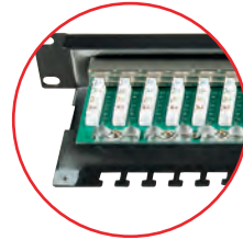
Face arrière !
